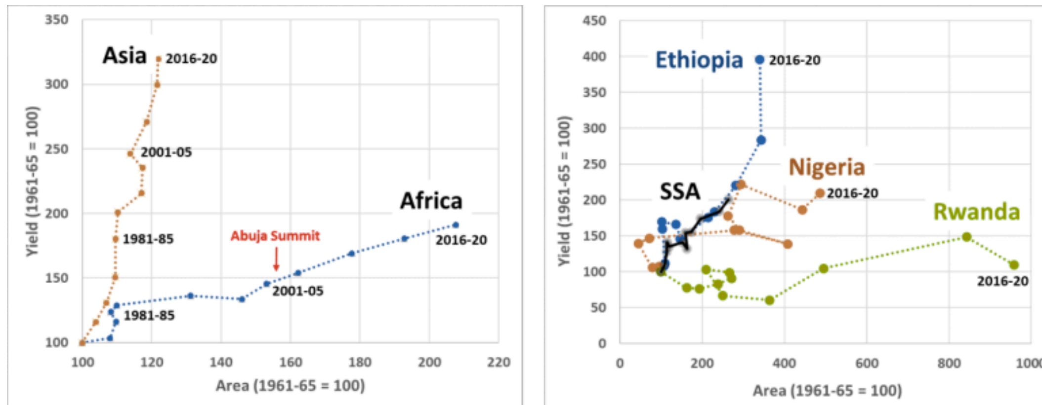
Abbildung 2. Relative Veränderungen im Getreideertrag und in der geernteten Fläche in Asien und Afrika (links) und im Maisertrag und in der Fläche in Sub-Sahara-Afrika (SSA), Äthiopien, Nigeria und Ruanda (rechts), 1961-2020. Die gezeigten Daten sind 5-Jahres-Durchschnitte, wobei der Durchschnitt von 1961-1965 als 100 gesetzt ist. Quelle: FAOSTAT .
