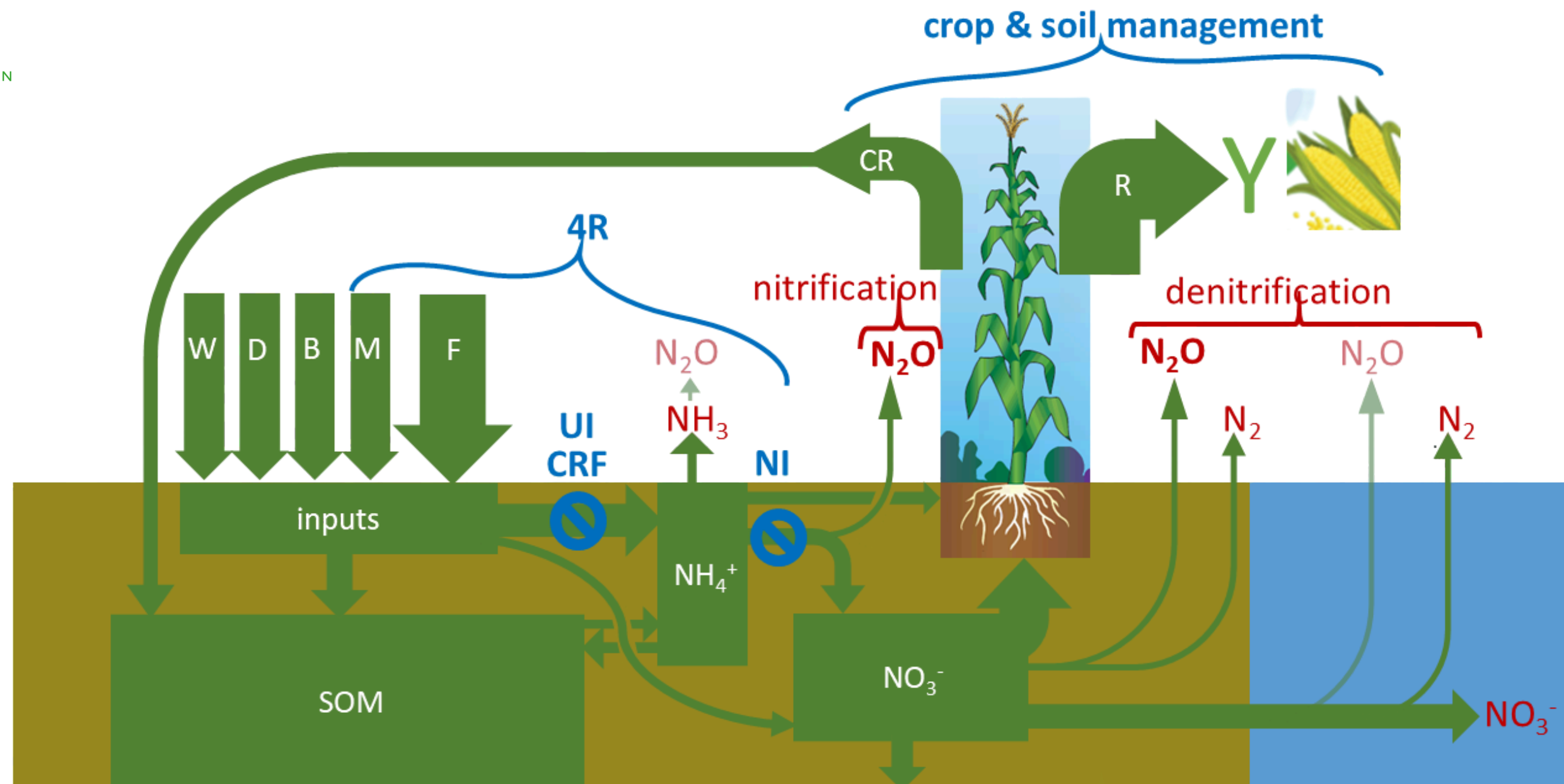
Abbildung 1. Quellen von N 2 O-Emissionen aus Stickstoff (N)-Einträgen in landwirtschaftliche Böden. Die Emissionen steigen bei der Ausbringung von Düngemitteln (F) oder Wirtschaftsdünger (M). Direkte Emissionen entstehen, wenn Ammonium (NH 4 + ) nitrifiziert und Nitrat (NO 3 - ) denitrifiziert werden. Indirekte Emissionen entstehen durch Verluste ins Abwasser und durch Ammoniak (NH 3 )-Verluste in die Luft. Zusätzliche Einträge umfassen die biologische Stickstofffixierung (B), atmosphärische Deposition (D) und Bewässerungswasser (W). Die Rückführung von Ernterückständen (CR) trägt ebenfalls N zu den Bodenpools hinzu, aus denen N 2 O emittiert wird. Die Optimierung der N-Nutzungseffizienz (NUE) – durch möglichst genaue Anpassung der Einträge an die Ernteabfuhr (R) – wird durch Management der Einträge (4R), Kulturen und Böden zur Optimierung der Erträge (Y) erreicht. Verbesserungen der NUE reduzieren die Düngemittlemissionen pro Einheit erzeugtes Produkt. Nitrifikationshemmer (NI), Dünger mit kontrollierter Freisetzung (CRF) und Ureasehemmer (UI) sind effektive 4R-Praktiken, die die N 2 O-Emissionen pro eingesetzte N-Einheit verringern.
