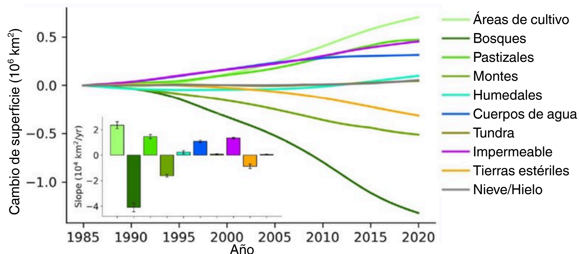
Figura 2. Cambios globales en el uso de la tierra desde 1985 (6). La tendencia muestra un aumento en el área de pastizales y tierras de cultivo mientras que disminuyen áreas de bosques y montes.
